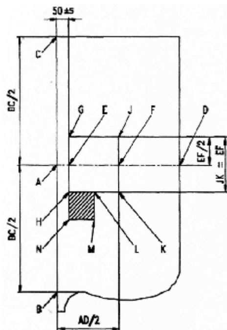
Rys. 3. Miejsca pobrania próbek pierwotnych z kruponów i półkruponów [PN-EN ISO 2418: 2005]
