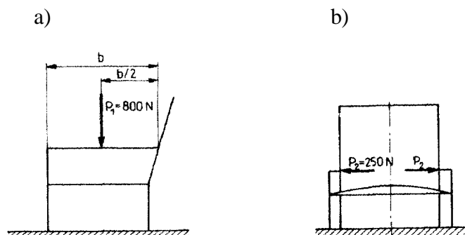
Rys. 27. a) badanie poręczy fotela na działanie siły pionowej, b) badanie poręczy fotela na działanie siły poziomej. [5, s 173]
