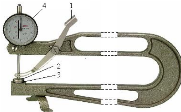
Rys. 8. Grubociomierz sprężynowy [25]: 1 – dźwignia, 2 – stopka czujnika ruchoma, 3 – stopka czujnika stała, 4 – licznik
