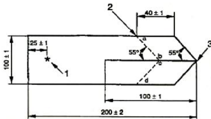
Rys. 19. Kształt i wymiary próbki do oznaczania wytrzymałości na rozdieranie [PN-EN ISO 13937-3: 2002]
