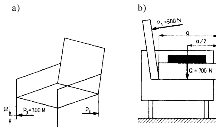
Rys. 28. a) badanie podstawy fotela, b) badanie oparcia fotela. [5, s 174]
