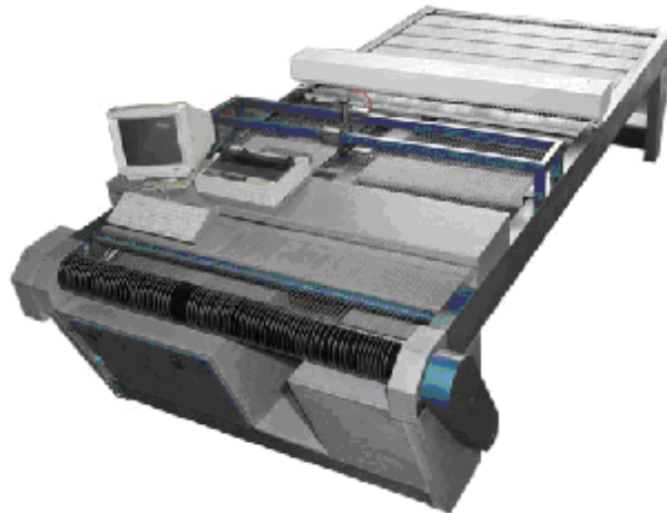
Rys. 7. Urządzenie elektroniczne do pomiaru powierzchni skór [18]
